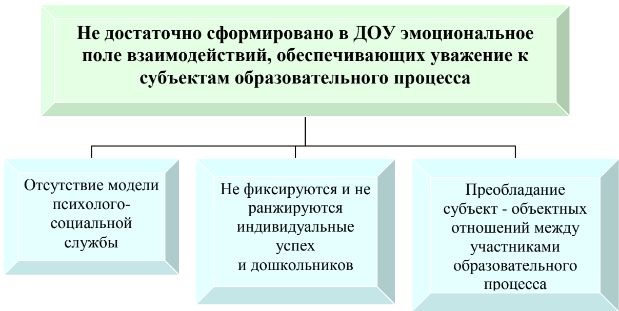
Рис. 41 Древо проблем
